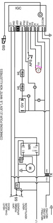
ELECTRICAL LADDER DIAGRAM / DIAGRAMME EN ESCALIER / DIAGRAMA ELECTROICO DE ESCALERA
